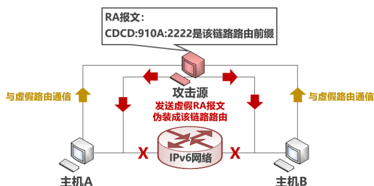
图 3.11 前缀欺骗攻击
