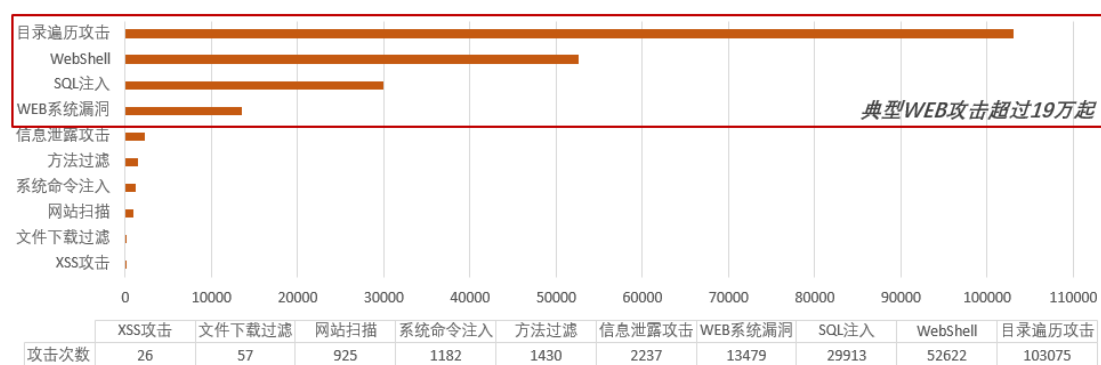
图 1.10 283 家云托管网站网络攻击情况
