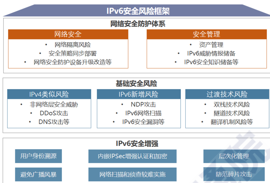
图 2.7 中国电信 IPv6 安全风险框架
