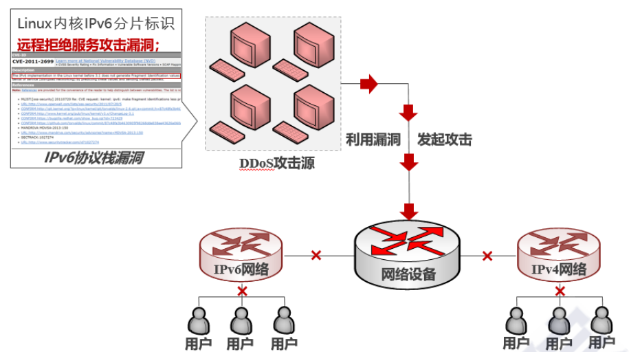
图 3.2 双栈机制安全风险
