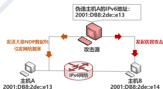
图 3.9 NDP 攻击
