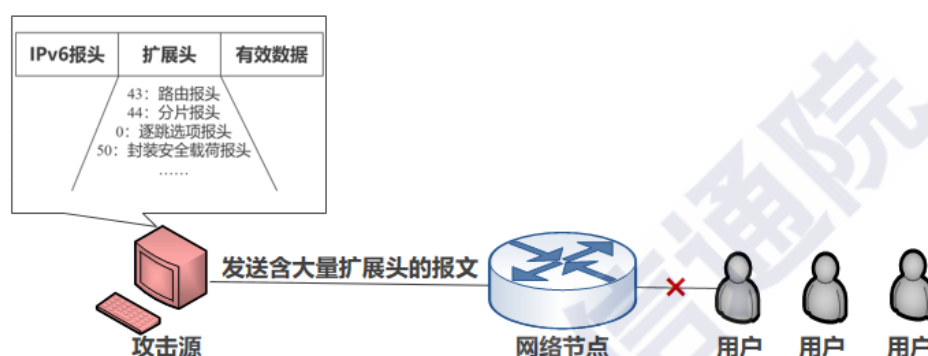
图 3.8 扩展头攻击
