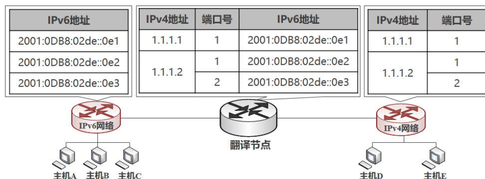
图 3.5 翻译机制原理
